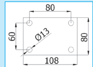
Podstawa mała / Small base
