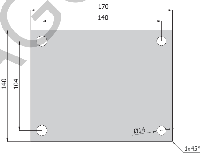
dotyczy obudów do pługów i zmiatarek do kół / for snowplough and roadsweeper housings with wheels \varnothing 250
