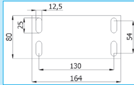
Podstawa duża / Large base
